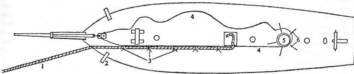
Manier van anker hieuen met behulp van een kabelaring. 1. ankerkabel; 2. kraanbalk; 3. seizings; 4. kabelaring (touw zonder eind); 5. gangspil; 6. windbomen of handspaken (n. Sp.)
